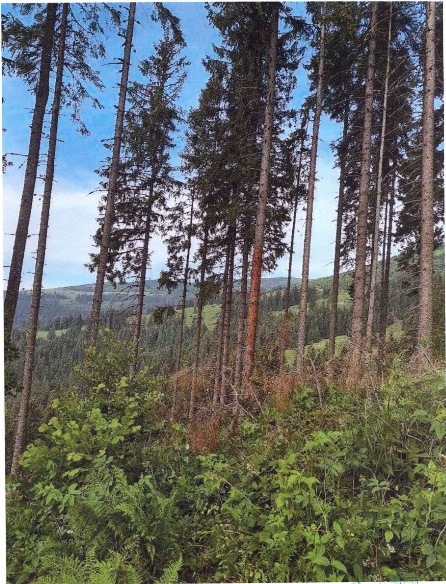
Fotografie cu arbori infestati de Ipsidae UPI, ua 15A
