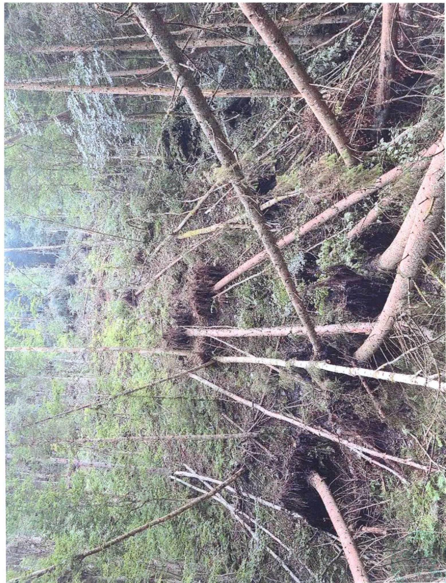
Fotografie cu arbori deformati de vânt , UP 1 , ua 39A
